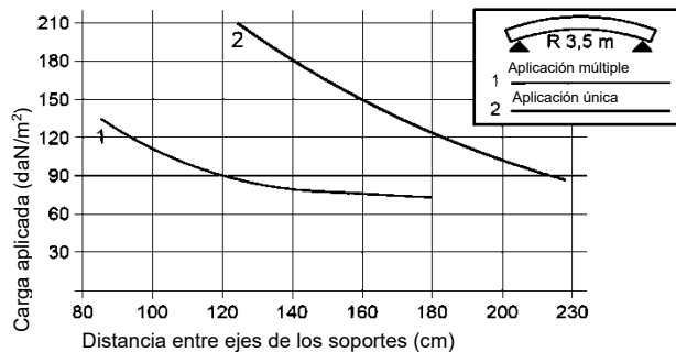
CARGAS GRECA 28/112 esp. 6 mm aplicación curva R3500 mm
