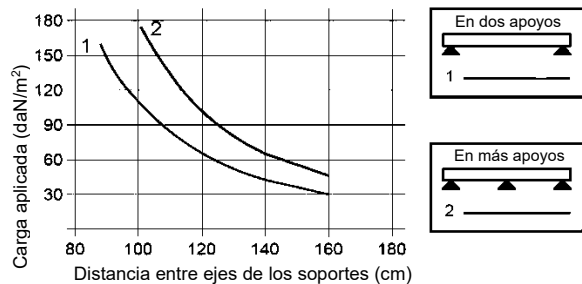
CARGAS GRECA 28/112 esp. 6 mm aplicación plana
